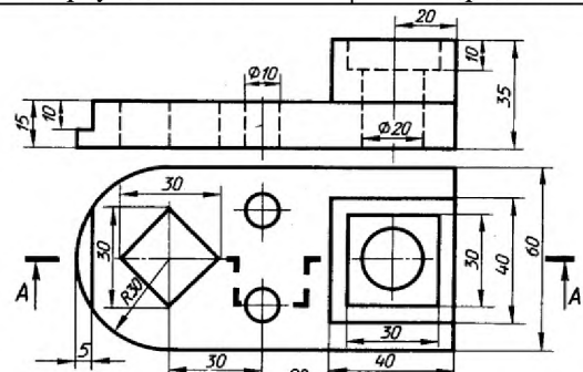
Корпус. Сталь 30.
