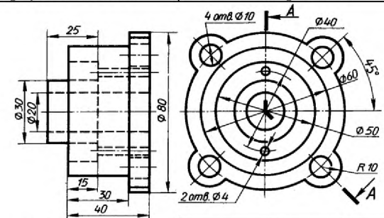
Фланец Чугун СЧ 15.
