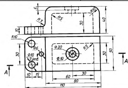
Корпус. Сталь Ст3.
