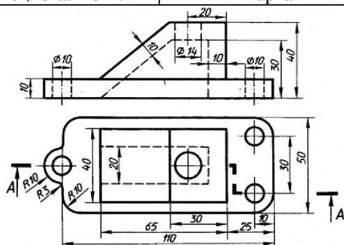
Корпус. Сталь 20.
