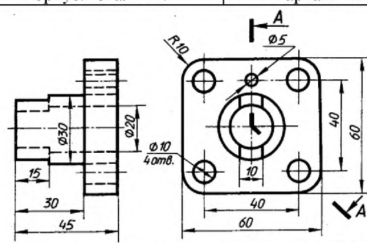
Фланец. Сталь 30.
