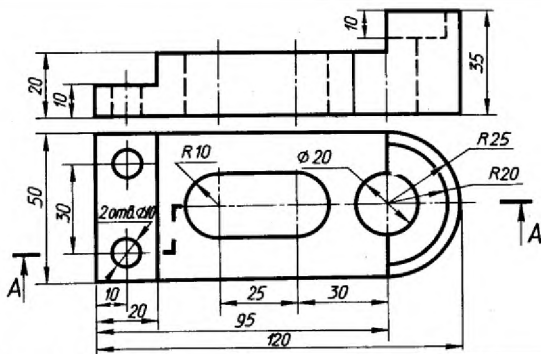
Корпус. Сталь 45.
