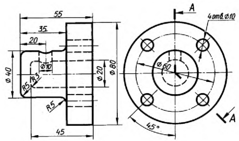
Корпус. Чугун СЧ 15.
