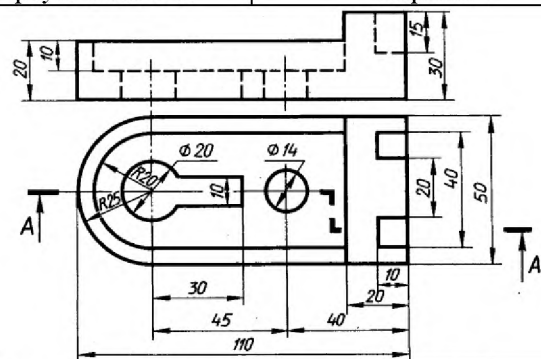
Корпус. Сталь Ст3.
