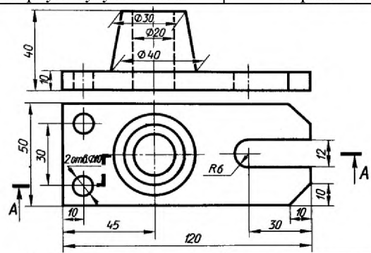
Корпус. Сталь 45.
