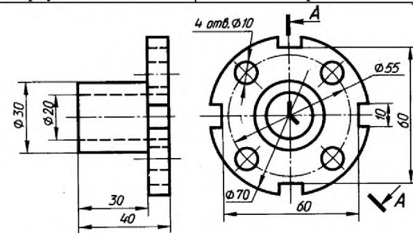
Фланец. Сталь Ст3.
